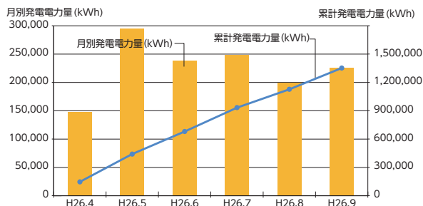
自社発電所 月別発電電力量
